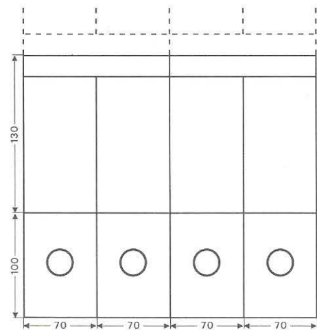
Anbau Rückseite Backside mounting
